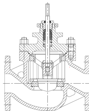
笼式单座型座阀
