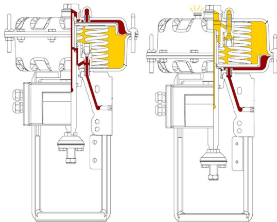
三断锁定型智能定位器
