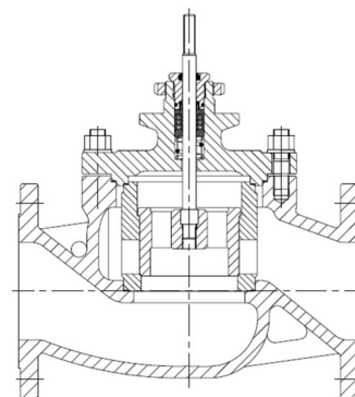
套筒式压力平衡型座阀
