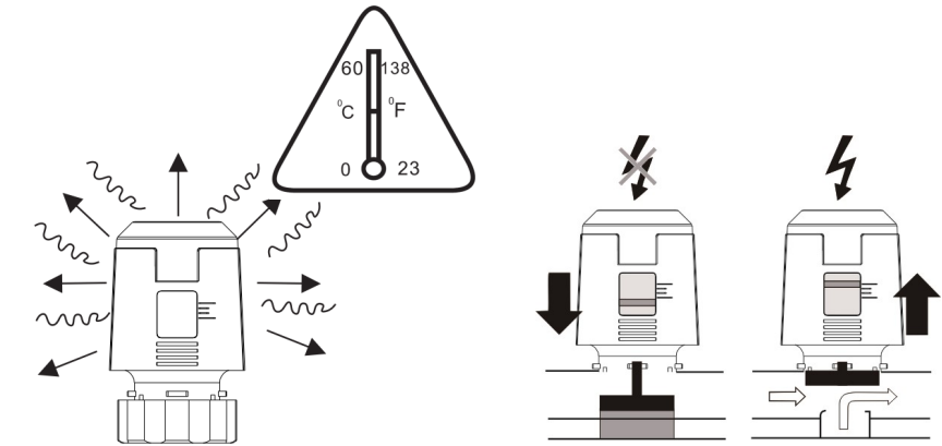
安装示意图
