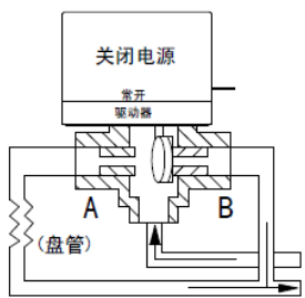
图 5：三通阀分流布置（常开）管道安装
