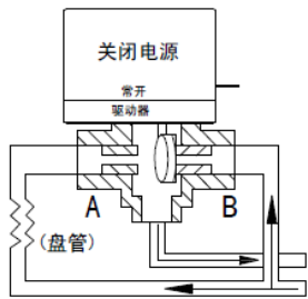
图 2：三通阀混合布置（常开）管道安装
