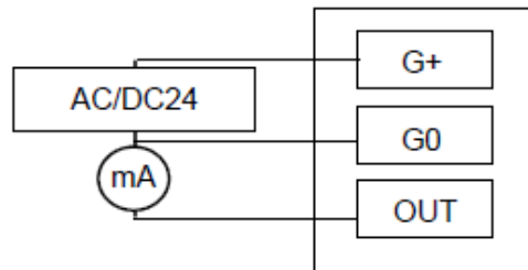
3 线制
