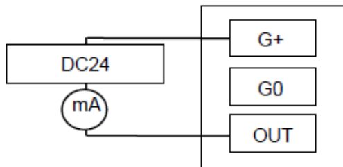
2 线制
